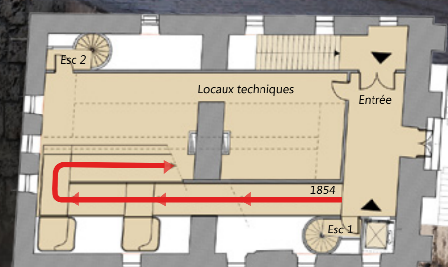
Plan RDC ech 1/200
